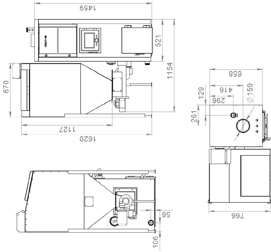
Пеллетный котел "СТАРТ-30-GR-V1", бункер 400 литров
